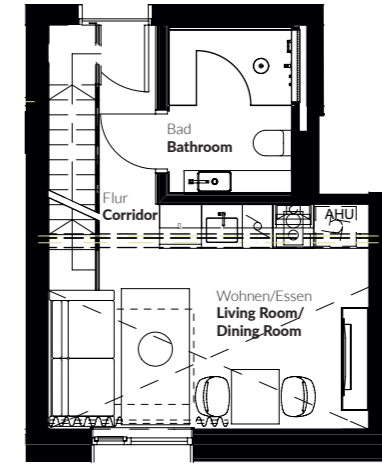
3.OG 3 rd floor
